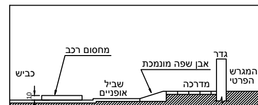
ירידה לכביש כאשר יש חניה ושביל אופניים
