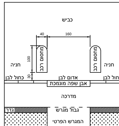
ירידה לכביש כאשר יש חניה
