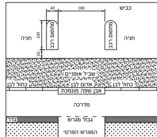
ירידה לכביש כאשר יש חניה ושביל אופניים
