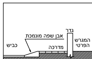
ירידה לכביש כאשר אין חניה
