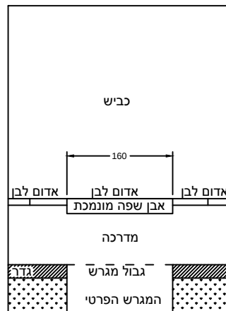
ירידה לכביש כאשר אין חניה
